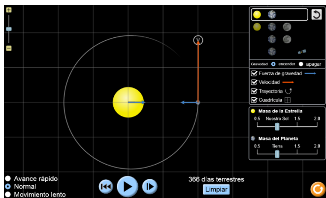
Figura 1: Sistema Tierra – Sol.
