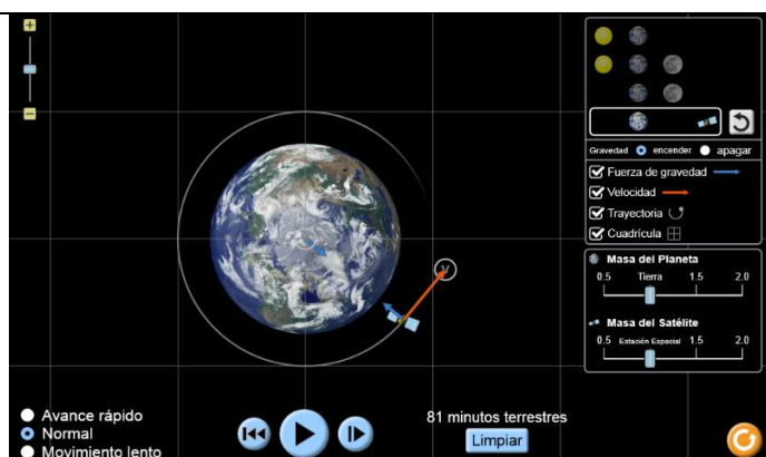
Figura 3: Sistema Tierra – satélite artificial
