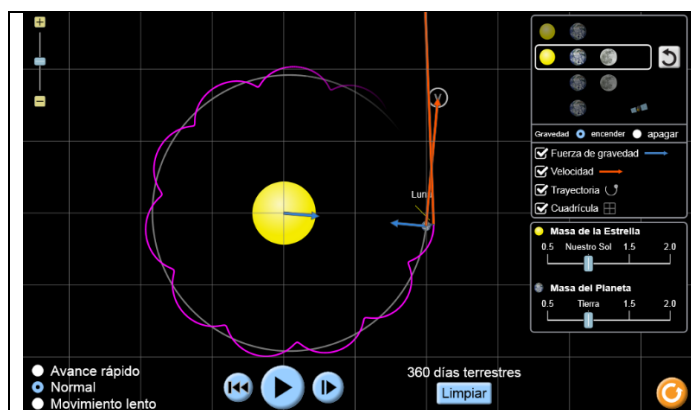
Figura 2: Sistema Sol – Tierra - Luna
